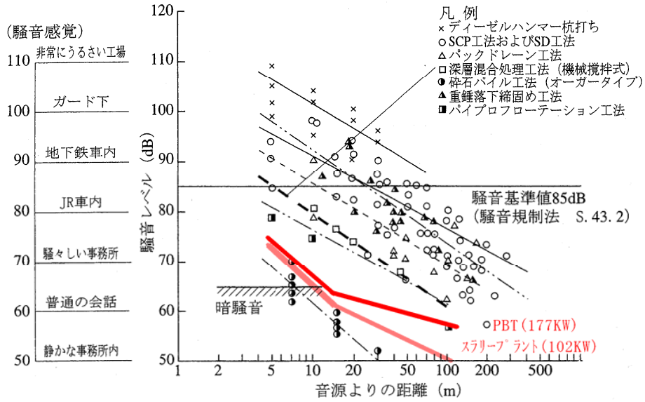
図-1 深層混合処理工法における騒音感覚、騒音レベルの距離減衰
