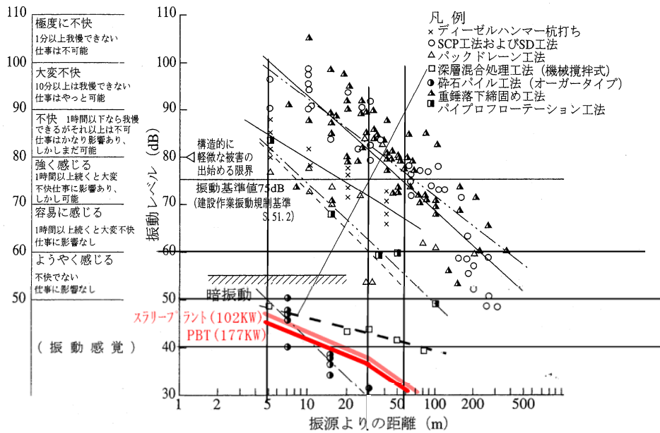
図-2 深層混合処理工法における振動感覚、振動レベルの距離減衰
